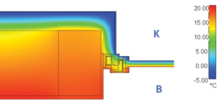
5. ábra: Ablakbeépítés csomópont hőmérséklet-eloszlásának számítógépes modellezése.
