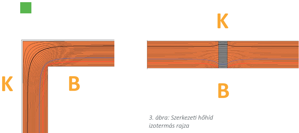
2. ábra: Geometriai hőhíd izotermás rajza
