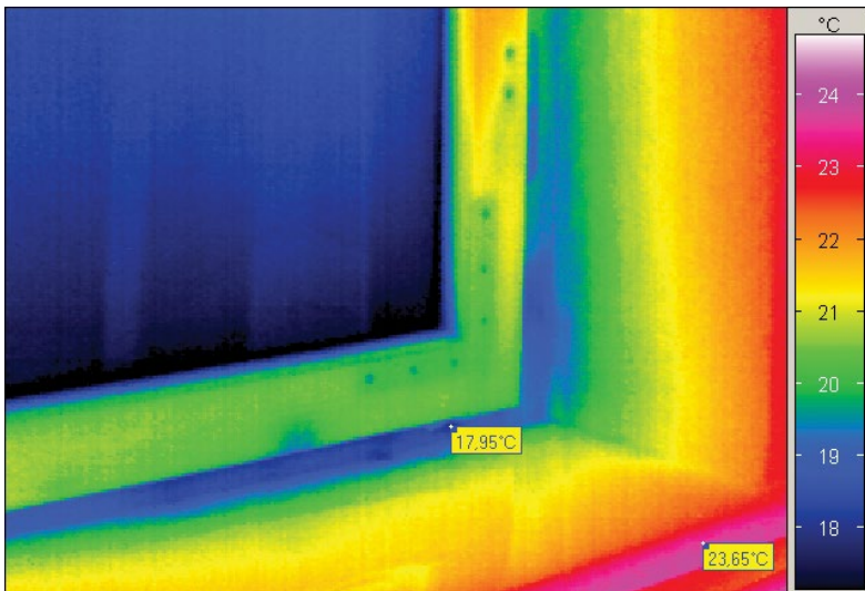
4. ábra: Jellegzetes hőmérséklet-eloszlás ablakkávéban (hagyományos ablak belső oldaláról készült hőfotó)
