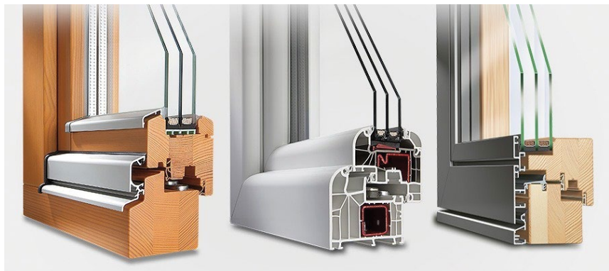
1. ábra: Különböző anyagú koszerű nyílászárók szerkezeti kialakítása
