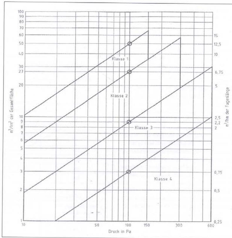
3. ábra. Légáteresztési osztályok az MSZ EN 12207:2001 alapján
