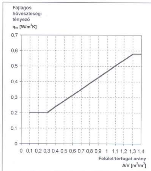
1. ábra. A fajlagos hővesztés-tényező követelményértéke
